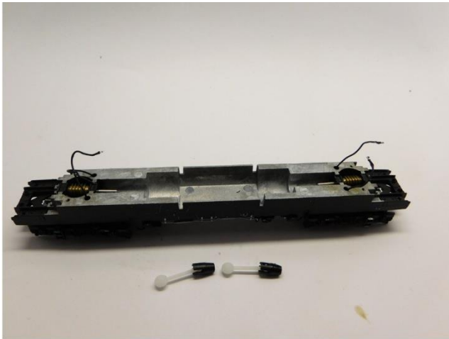
Ausbau alter Kardankupplungen Take out old cardan couplers Demonteer de cardan koppelingen
