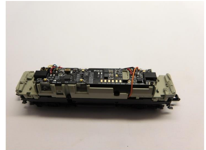
Rahmen und Platine platzieren Mount frame and PCB Plaats het frame en de printplaat
