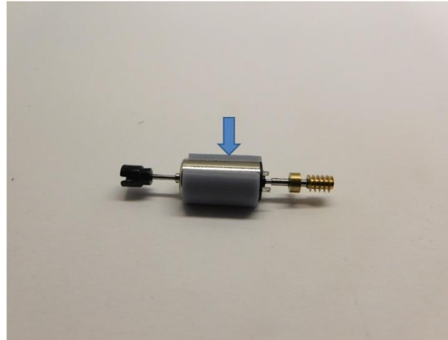
Der Motor wird mit Epoxidkleber oder Sekundenkleber in den Motorhalterteile eingeklebt The motor is glued into the motor holder parts with epoxy glue or super glue
