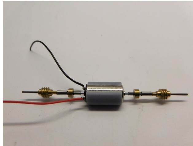
Kleben Sie die Wellen Glue the axles Verlijm de assen
