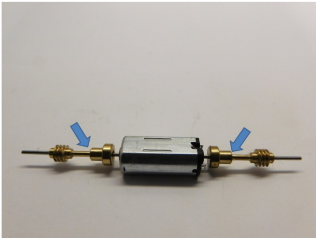
Die Wellen mit einer Trennscheibe kürzen Cut the axles with a cutting disc De assen worden met een doorslijpschijf afgeslepen
