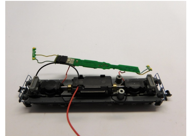
Motorhalter und die Drehgestellabdeckungen platzieren Mount motor holder and bogie covers Motorhouder en draaistel afdekkingen monteren
