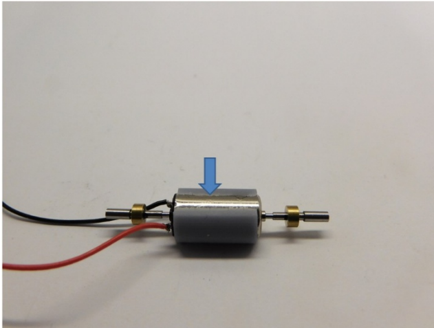
Der Motor wird mit Epoxidkleber oder Sekundenkleber in den Motorhalterteile eingeklebt The motor is glued into the motor holder parts with epoxy glue or super glue De motor wordt in de motor houder delen verlijmd met secondelijm of epoxy lijm
