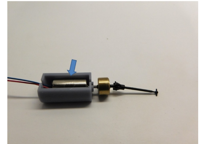
Der Motor wird mit Epoxidkleber oder Sekundenkleber in den Motorhalter eingeklebt The motor is glued into the motor holder with epoxy glue or super glue De motor wordt in de motor houder verlijmd met secundelijm of epoxy lijm
