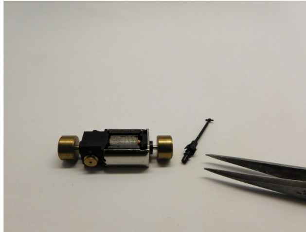
Sie brauchen dieses Teil wieder. Diese wird mit einer Pinzette entfernt You need the part again. It can be removed with tweezers U heeft het onderdeel weer nodig. Het wordt met een pincet verwijderd
