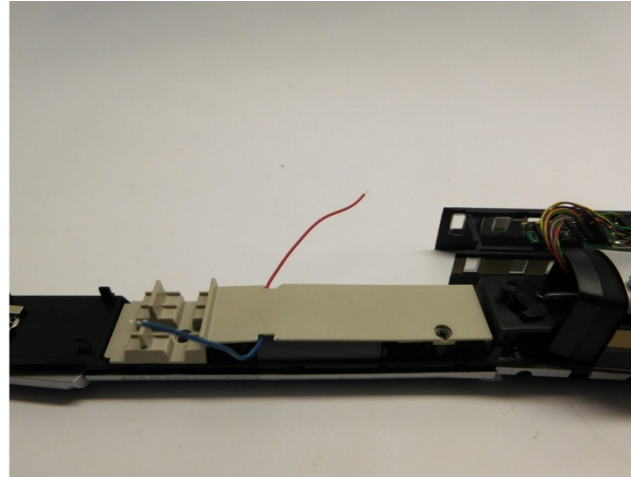
Abdeckplatte platzieren Mount cover plate Plaats de afdekplaat
