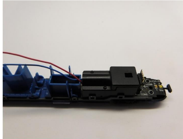
Motorhalter platzieren Place motor holder Plaats de motor houder
