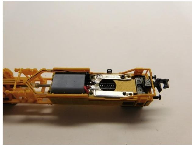
Platine platzieren Place PCB Plaats de printplaat
