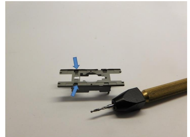
Bohren Sie 1.5 mm Löcher Drill 1.5 mm holes Boor gaten van 1.5 m
