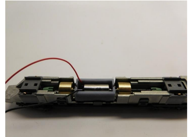
Platzieren der Motor in die Motorhalter Place the motor in the motor holder Plaats de motor in de motor houder
