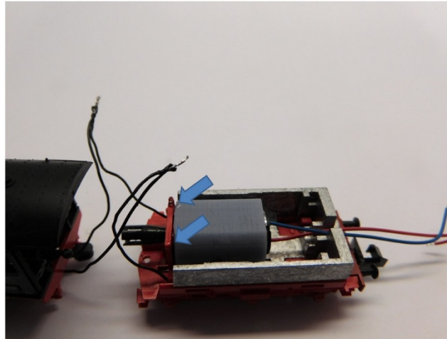
Kleben Sie den Motor Glue the motor Verlijm de motor
