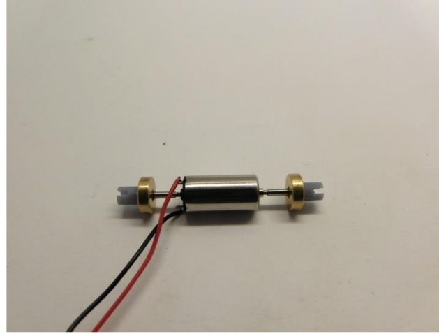
Die Teile sind geklebt The parts are glued De onderdelen zijn verlijmd
