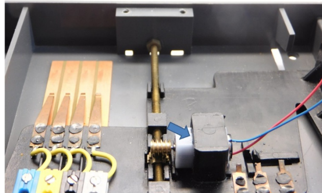
Motor kleben Glue the motor Verlijm de motor
