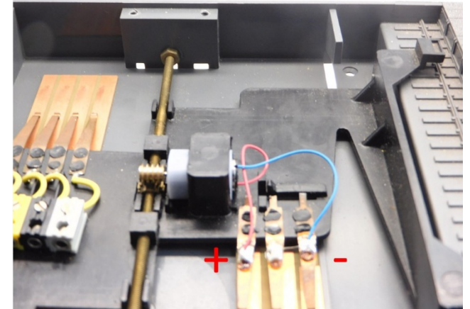
Löten Sie die Drähte Solder the wires Soldeer de draden
