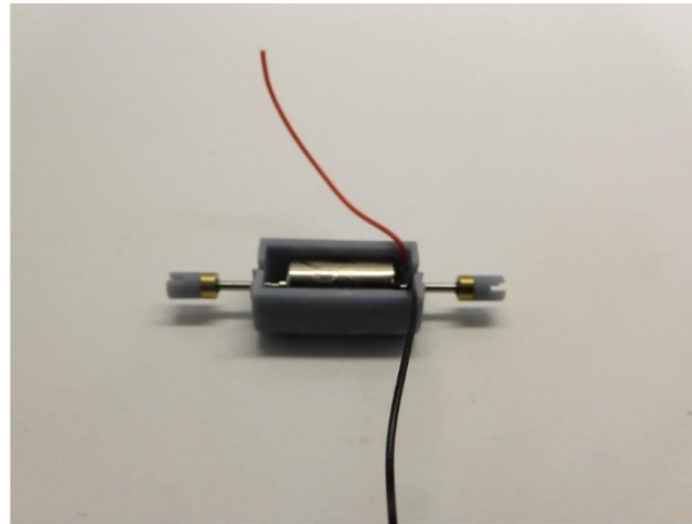
Kardankupplungshalter kleben Glue cardan coupler shafts Verlijm de cardan koppelingshouders
