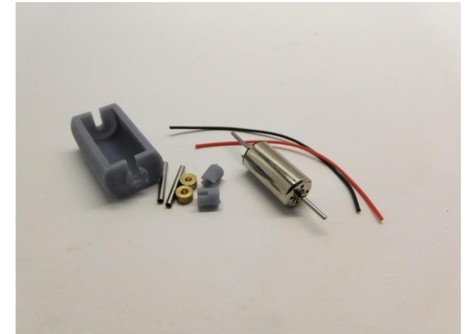
Die Teile des Bausatz The parts of the kit Onderdelen van de ombouwset
