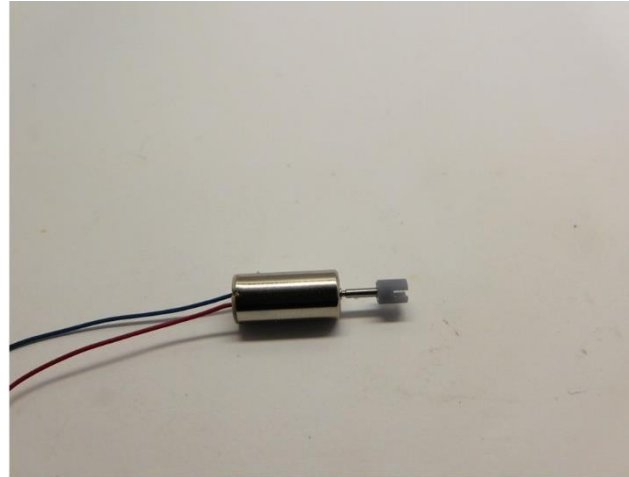
Kardankupplung platzieren Mount the cardan coupler Plaats de kardan koppeling
