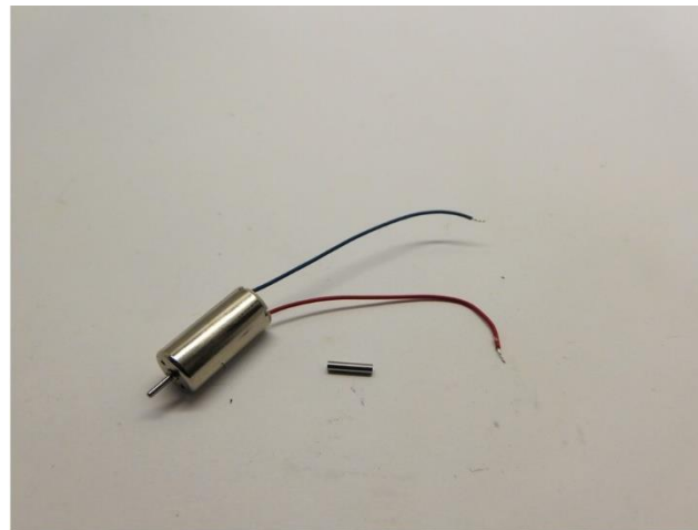
Die Metallteile werden mit Loctite oder Metall Epoxy kleber verklebt The metal parts are glued with loctite or metal epoxy glue Metalen onderdelen worden gelijmd met metaallijm of epoxylijm voor metalen
