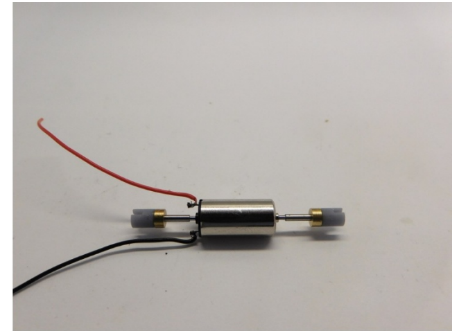
Kardankupplungen platzieren Mount the cardan couplers Monteer de kardankoppelingen
