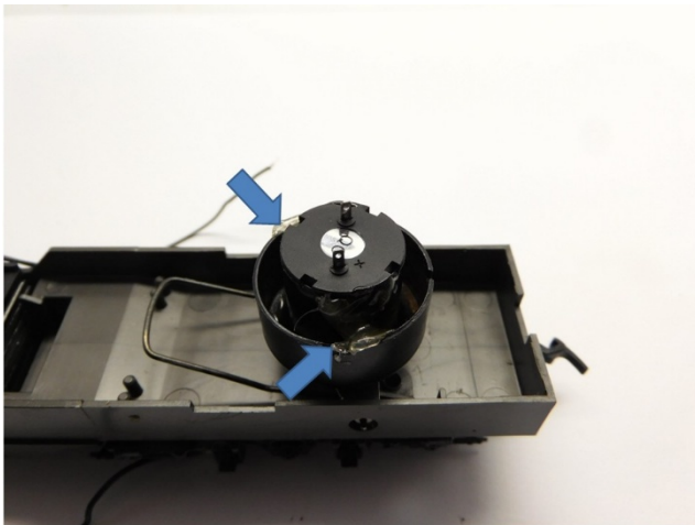
Der Motor wird mit Heizkleber geklebt The motor is glued with hotmelt De motor wordt met smeltlijm verlijmd
