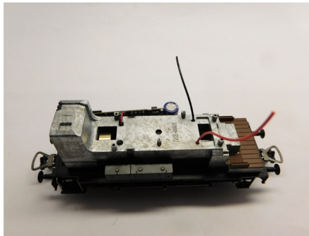
Gewicht platzieren Mount weight Gewicht plaasten
