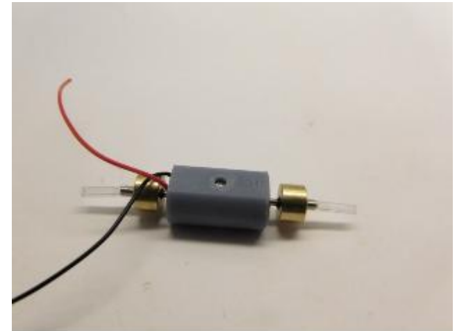
Schlauchkupplungen kleben Glue hose couplings Verlijm de slangkoppelingen
