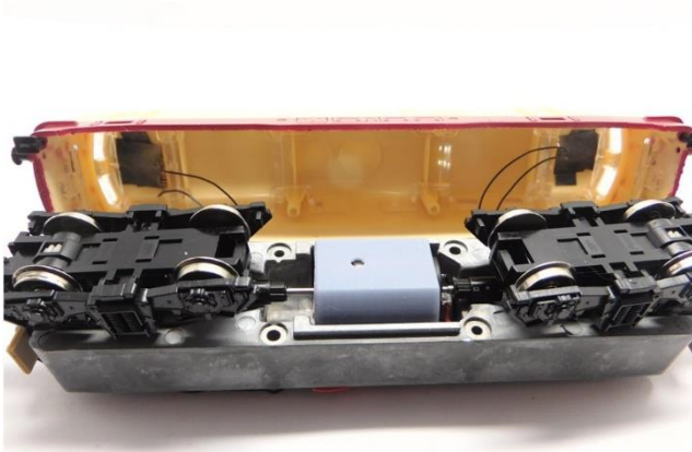
Motor platzieren Place the motor Plaats de motor
