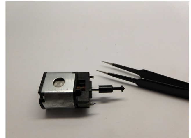
Sie brauchen die Teile wieder. Diese werden mit einer Pinzette entfernt You need the parts again. They can be removed with tweezers Je hebt deze onderdelen wederom nodig. Je kunt ze met een pincet verwijderen
