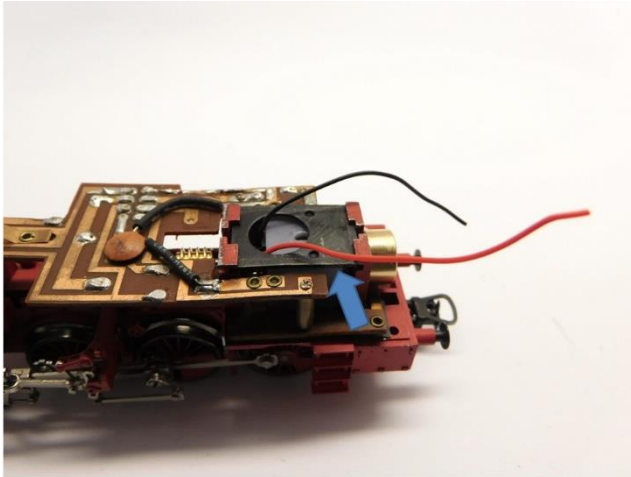
Motorhalter platzieren Mount motor holder Monteer de motorhouder
