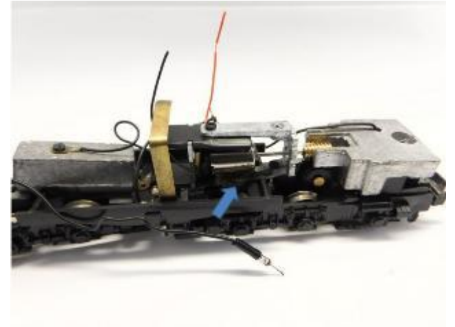
Motor kleben mit Heißkleber Glue the motor with hotmelt Lijm de motor met smeltlijm
