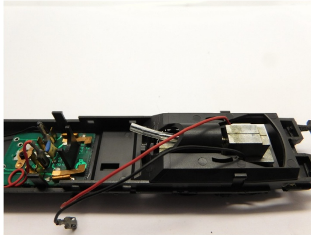
Schlauchkupplung kleben Glue the hose coupling Verlijm de slangkoppeling
