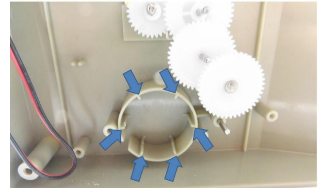
Material muss entfernt werden Material must be removed Materiaal moet verwijderd worden
