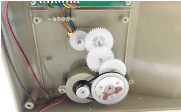
Motor platzieren Place the motor Plaats de motor
