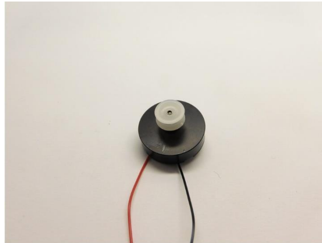
Riemenscheibe kleben Glue the pulley Verlijm de poelie
