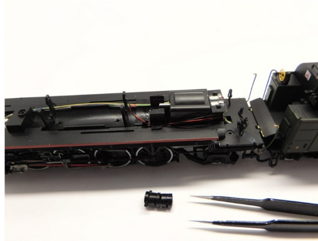
Ausbau Kardankupplung Take out cardan coupler Verwijder de kardankoppeling
