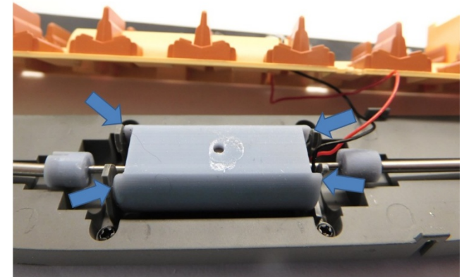
Der Motor wird geklebt The motor is glued De motor is verlijmd
