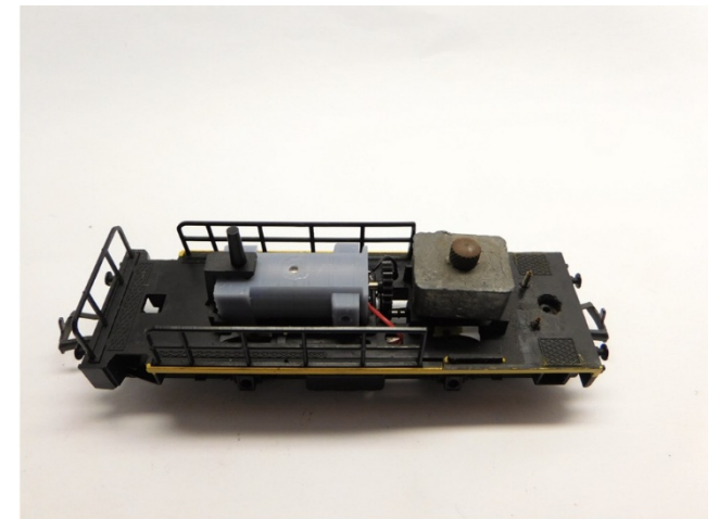
Motor platzieren Place the motor Plaats de motor
