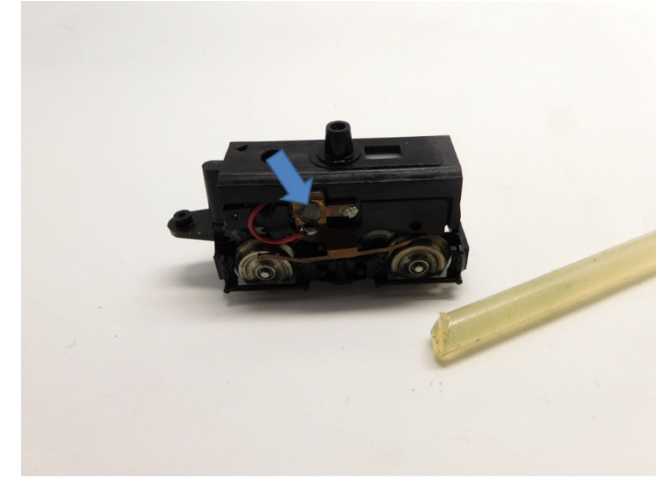
Kontakte kleben (Heizkleber) Glue contacts (Hotmelt) Verlijm de contacten (smeltlijm)
