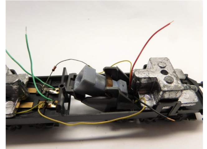
Schnecke platzieren Mount the worm gear Plaats het wormwiel
