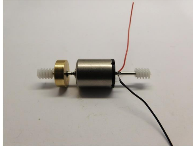
Schnecken kleben Glue worm gears Verlijm de wormwielen
