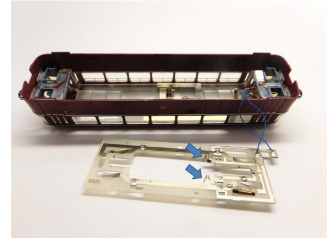
Alter Motorkontakt entfernen Remove old motor contacts Verwijder de oude motorcontacten
