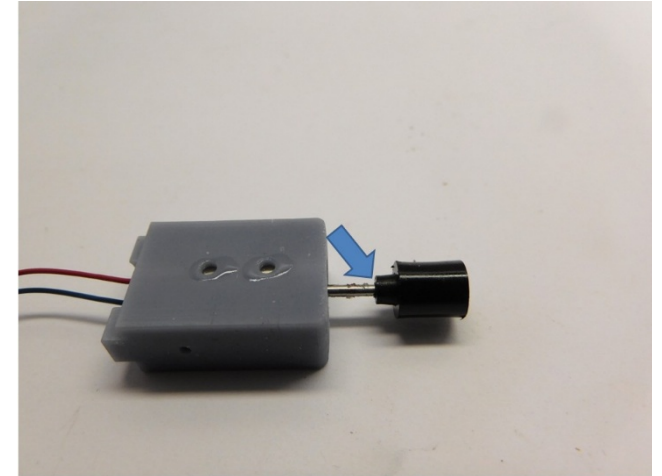
Kardankupplungshalter kleben Glue cardan coupler pocket Verlijm de cardankoppelingshouder
