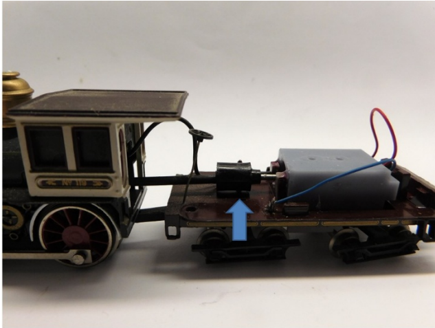
Raum prüfen Check clearance Controleer de speling
