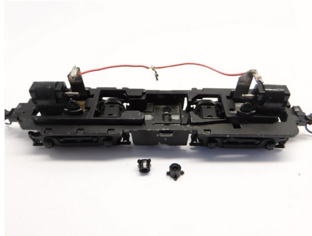
Entfernen Sie die Kardankupplungen Remove the cardan shafts Verwijder de cardan koppelingen
