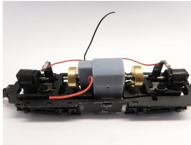
Motor prüfen Test fit the motor Controleer de passing
