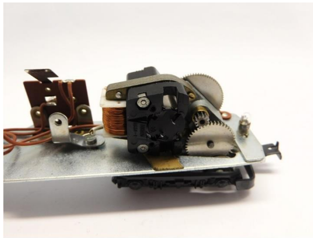
Motor kann mit einem Decoder oder Uhlenbrock FRU Fahrtrichtungsumschalter betrieben werden Motor can be used with a Decoder or an Uhlenbrock FRU
